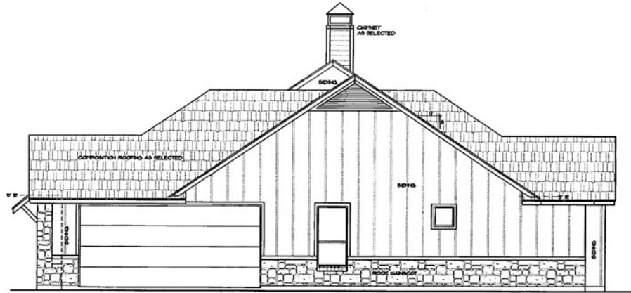
RIGHT ELEVATION
